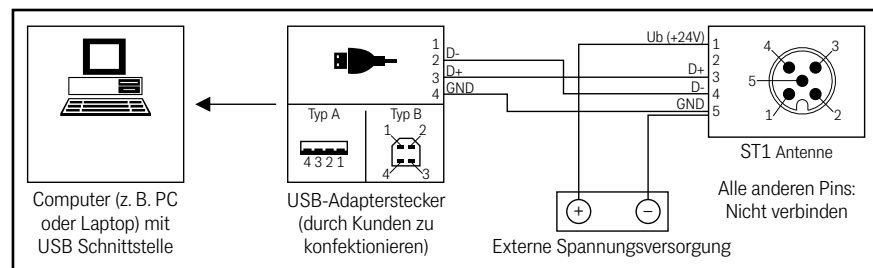
Bild 18 Anschlussbeispiel USB Verbindung mit der Schnittstelle eines PCs
