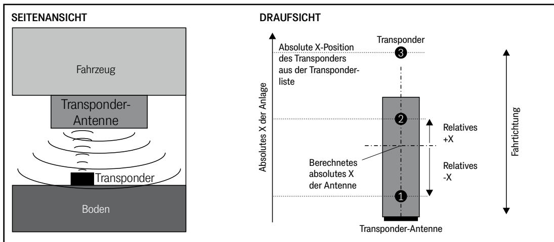
Bild 7 Skizze: Positionserkennung mit Transpondern
