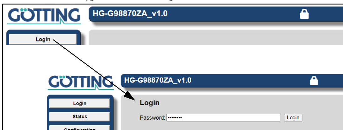
Bild 22 Konfigurations-Webseiten: Login
