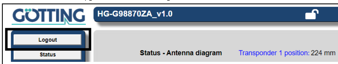
Bild 23 Konfigurations-Webseiten: Logout
