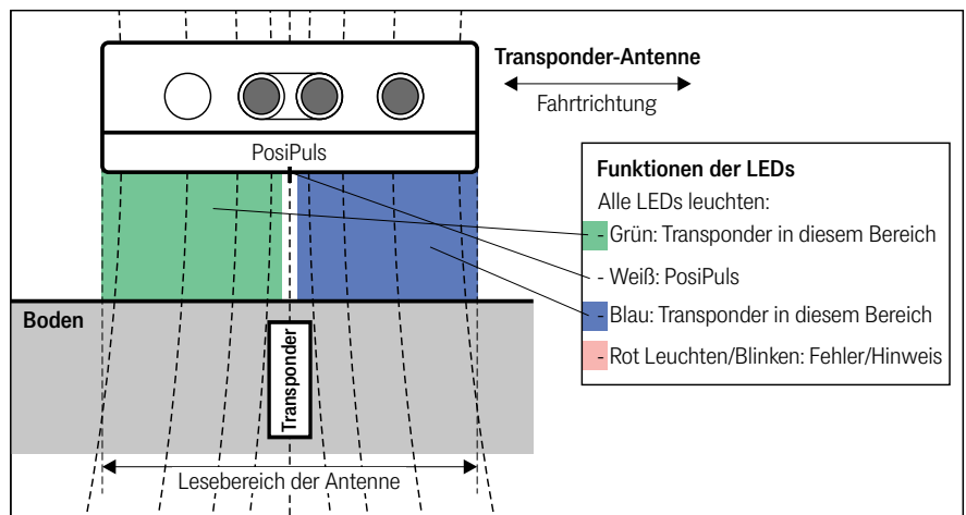
Lesebereich, PosiPuls und Funktion der LEDs
